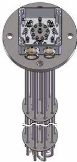
Flanschheizkörper flange heater
