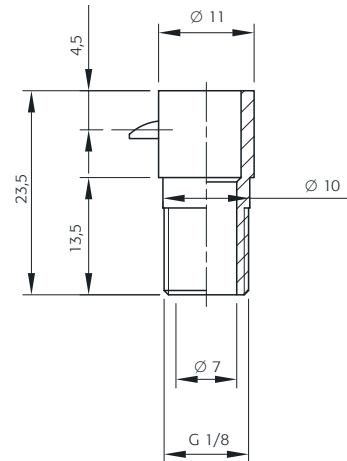
Nippel N4 Ø 11 mm G1/8 Nipple N4 Ø 11 mm G1/8
