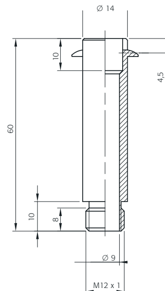
Nippel EN 32 Ø 14 mm L 60 mm M12x1 Nipple EN 32 Ø 14 mm L 60 mm M12x1
