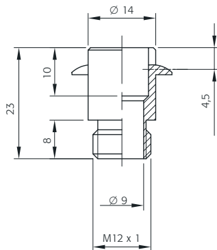
Nippel EN 32 Ø 12 mm L 23 mm M12x1 Nipple EN 32 Ø 12 mm L 23 mm M12x1
